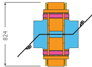
H - PILES
