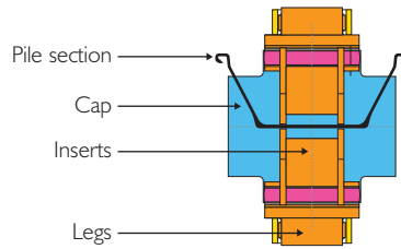
AZ - PILES SINGLY
